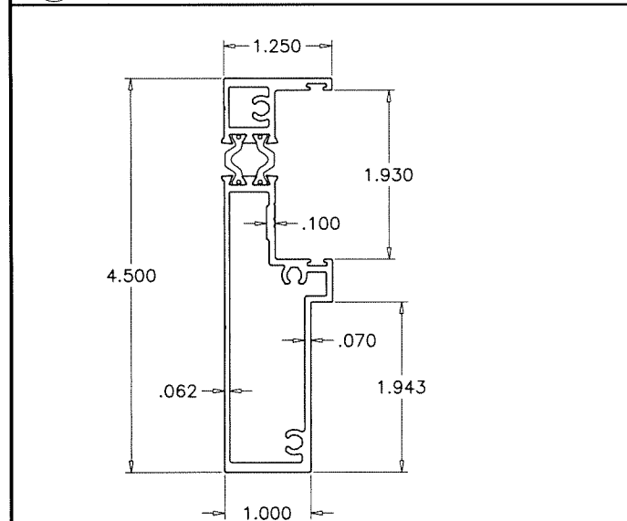
E2 FRAME JAMB
