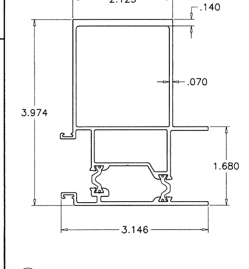
E11 ASTRAGAL STILE
