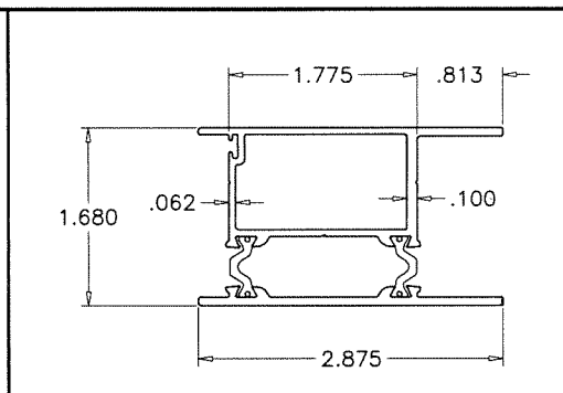
E4 JAMB STILE
