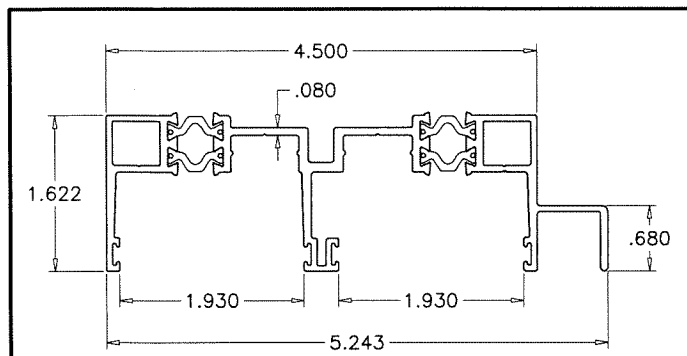
E1 FRAME HEAD
